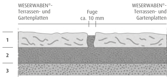
Abb. 1: Prinzip-Skizze Terrassenplatten Opus und Solum
